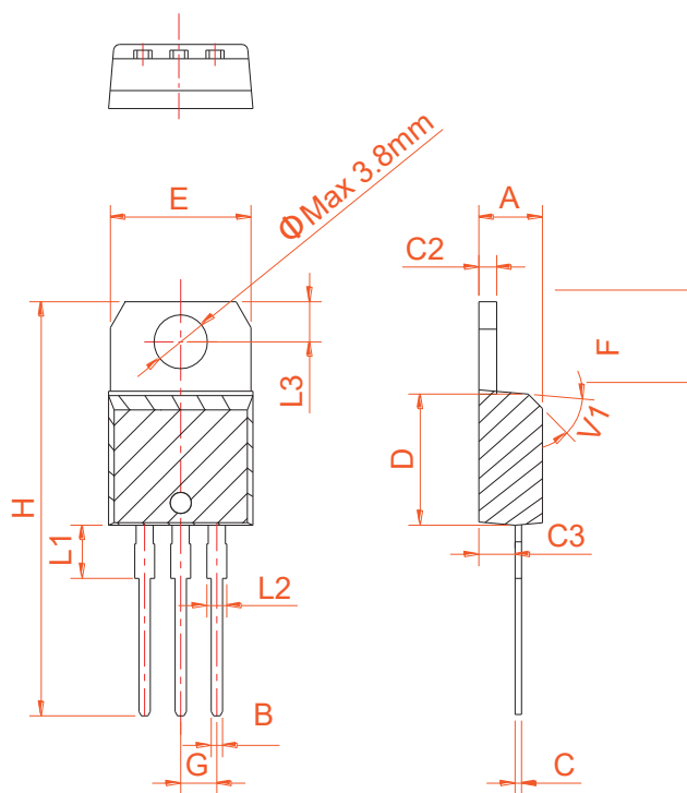
TO-220A Ins
